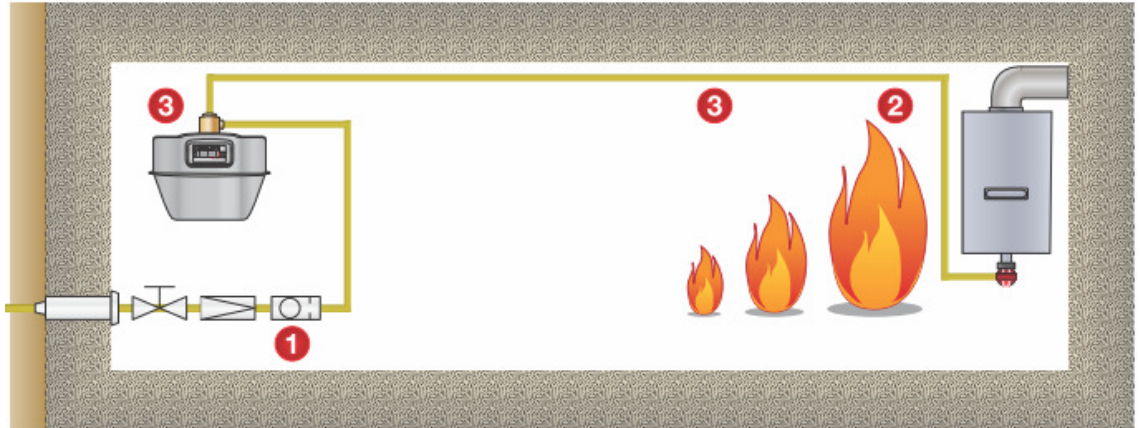
Bild 6 Prinzip der dreistufigen Sicherheitskette für Kunststoffrohre in der Gashausinstallation nach TRGI 2008
